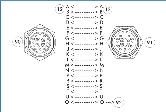
12 Masterzijde 91 M16-aansluiting, 19-polig 13 Adapterzijde 92 leidpin 90 M16-connector, 19-polig
