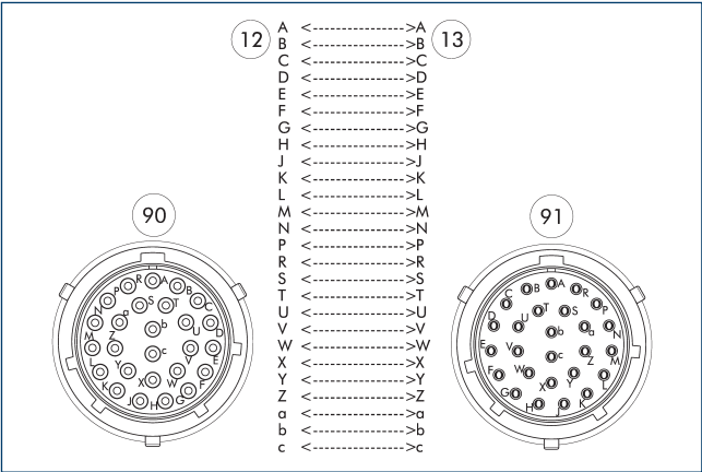
12 Masterzijde 13 Adapterzijde 90 Amphenol PT bajonetsluiting connector, 26-polig 91 Amphenol PT bajonetsluiting aansluiting, 26-polig
